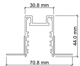
Profilo
